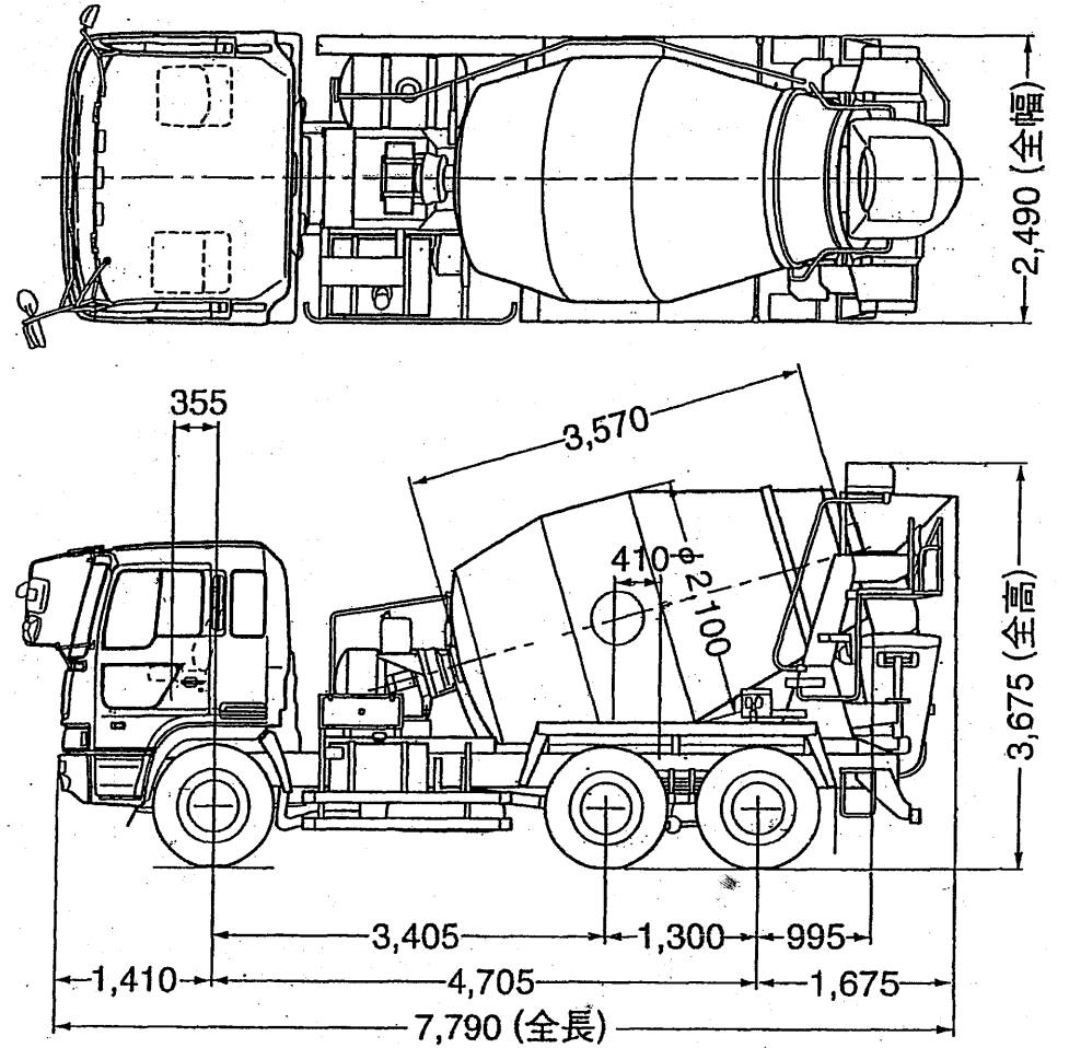
10 t ミキサー車
